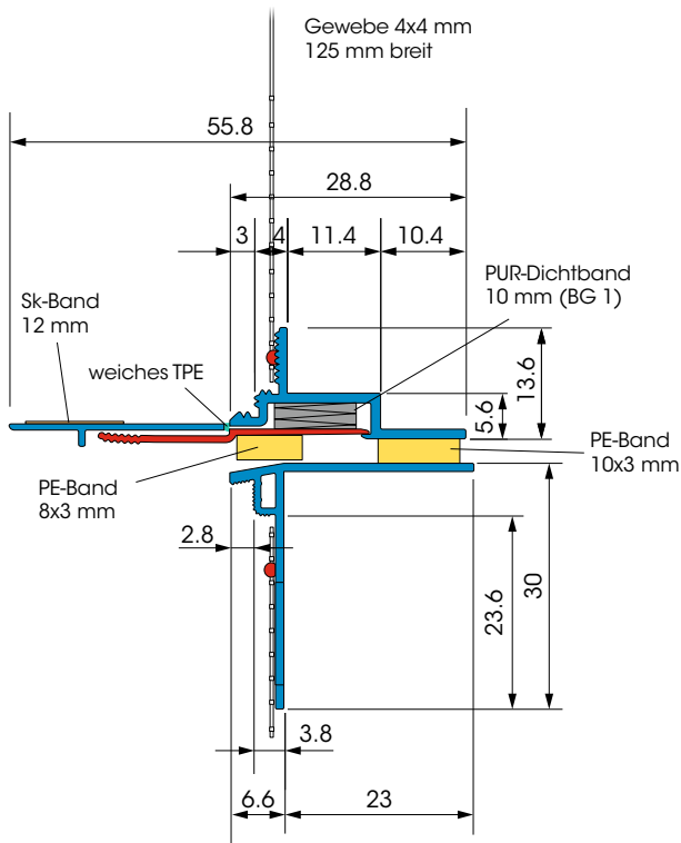
Schnittzeichnung in mm
