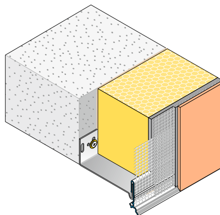
Anwendungszeichnung
