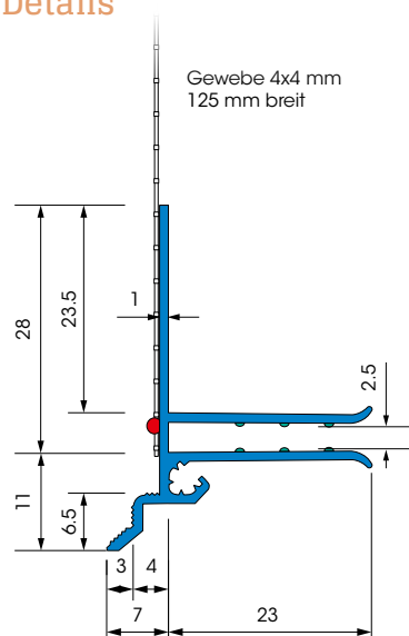
Schnittzeichnung in mm
