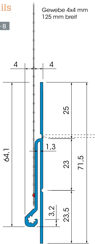
Schnittzeichnung in mm
