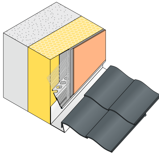
Anwendungszeichnung
