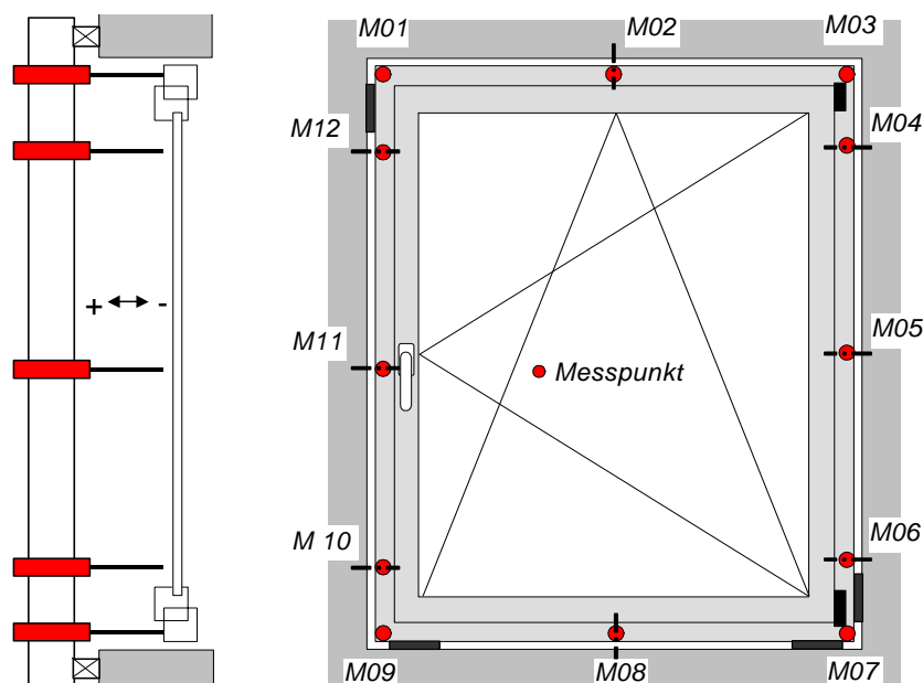
Bild 5 Schematische Darstellungen der Position der Befestigungspunkte und der Linearpotentiometer
