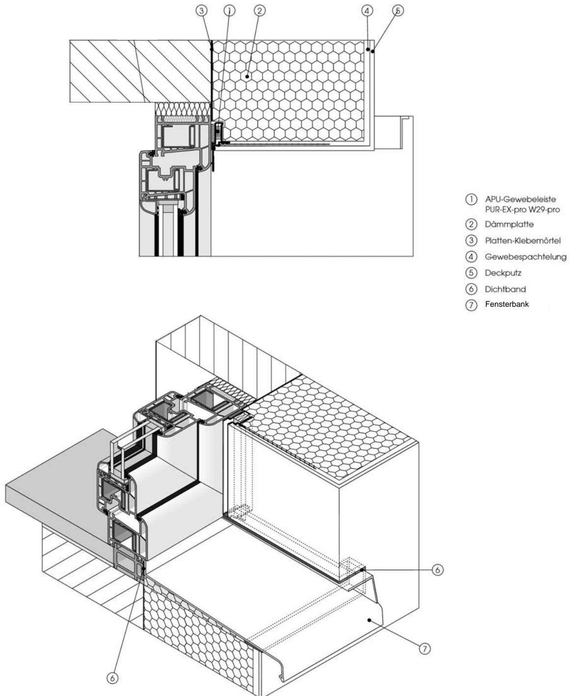
Abbildung 1 Außenseitiger Baukörperanschluss mit W29-pro APU Gewebeleiste PUR-EX-pro.
