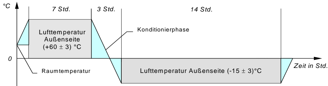
Abbildung 6 Darstellung der Temperatur-Wechselbelastung für einen Zyklus
