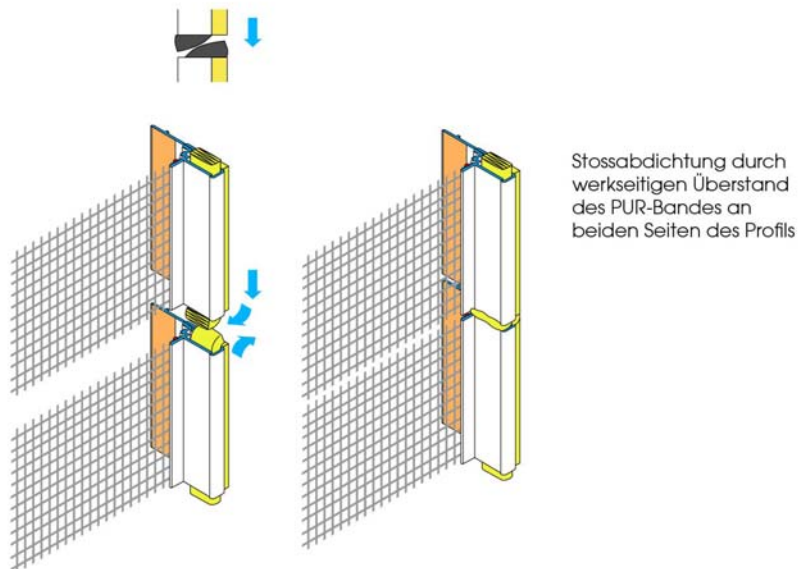
Abbildung 4 Längsstoßausbildung W29-pro APU Gewebeleiste PUR-EX-pro, Variante C
