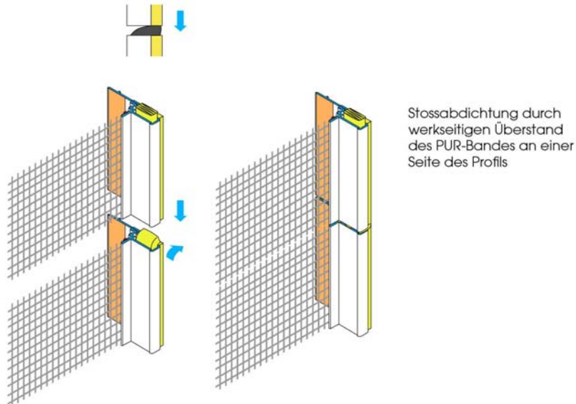
Abbildung 3 Längsstoßausbildung W29-pro APU Gewebeleiste PUR-EX-pro, Variante B
