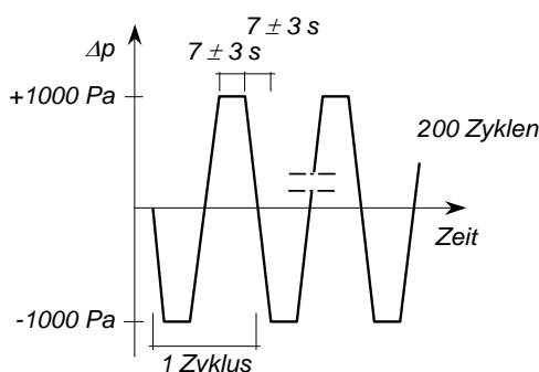
Abbildung 7 Darstellung der Druck-Sog-Wechselast
