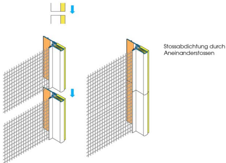
Abbildung 2 Längsstoßausbildung W29-pro APU Gewebeleiste PUR-EX-pro, Variante A
