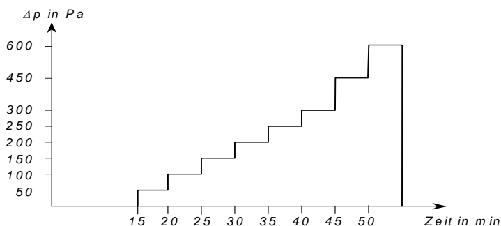
Abbildung 5 Darstellung der Druckstufen und des zeitlichen Verlaufes
