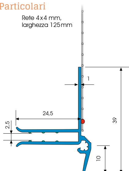
Sezione in mm
