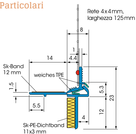
Sezione in mm
