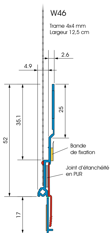
Plan de coupe en mm
