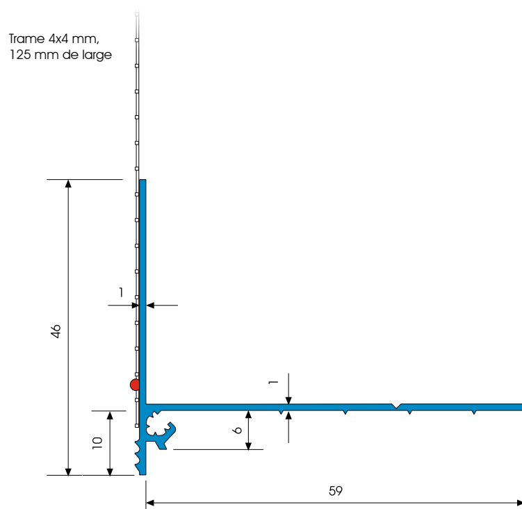
Plan de coupe en mm
