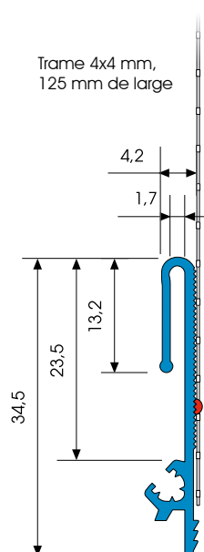
Plan de coupe en mm
