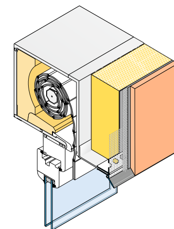
Schéma d'application 3D
