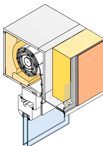
Schéma d'application 3D
