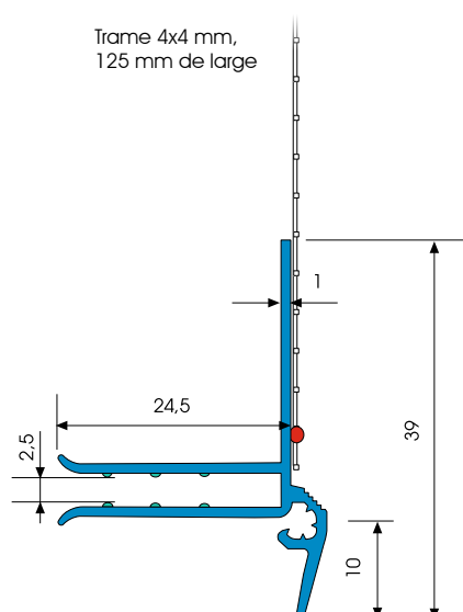
Plan de coupe en mm
