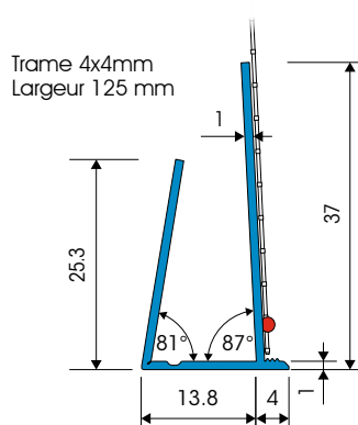
Schéma en coupe en mm
