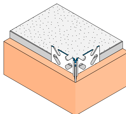
Schéma d'application
