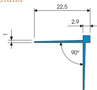
Schéma en coupe en mm
