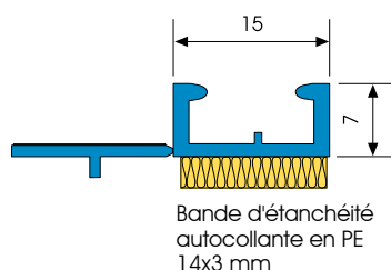
Plan de coupe en mm
