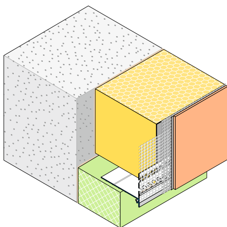
Dibujo de aplicación
