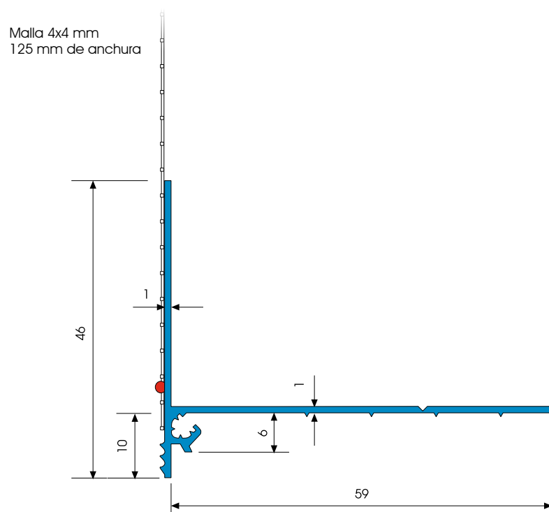
Dibujo seccional en mm
