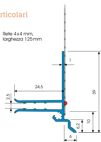
Sezione in mm
