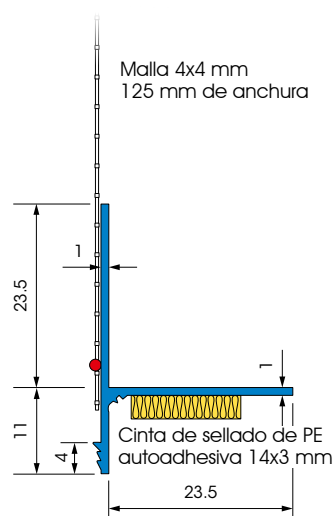
Dibujo seccional en mm
