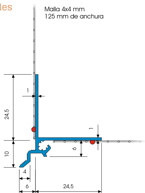
Dibujo seccional en mm
