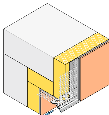
Dibujo de aplicación
