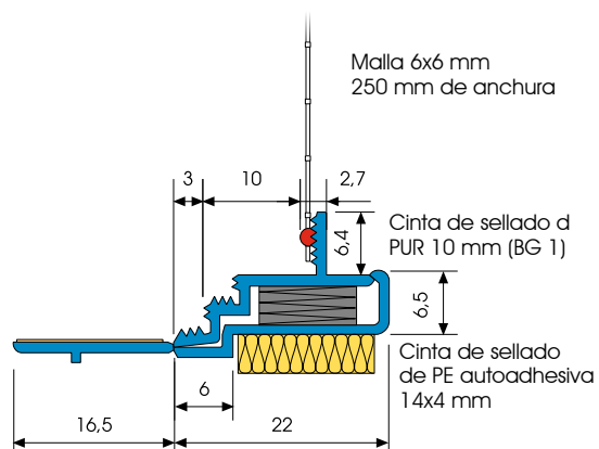
Dibujo seccional en mm
