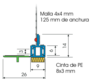
Dibujo seccional en mm
