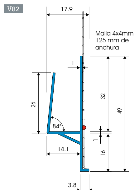
Dibujo seccional en mm
