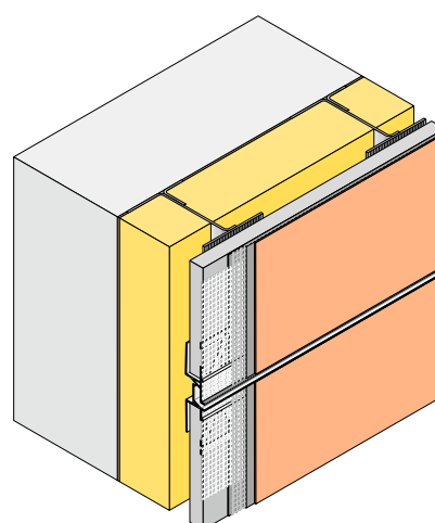
Dibujos de aplicación
