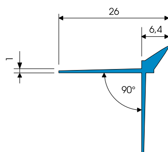
Dibujo seccional en mm
