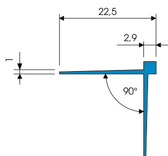
Dibujo seccional en mm
