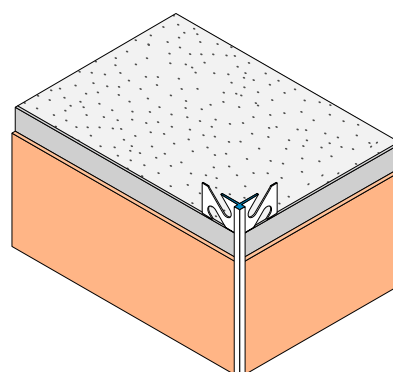
Dibujo de aplicación
