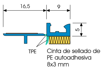
Dibujo seccional en mm
